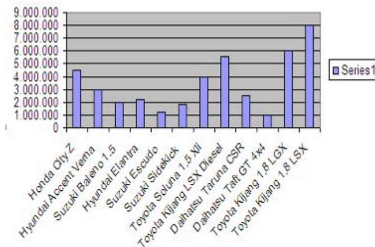
Gambar 36. Grafik kolom
