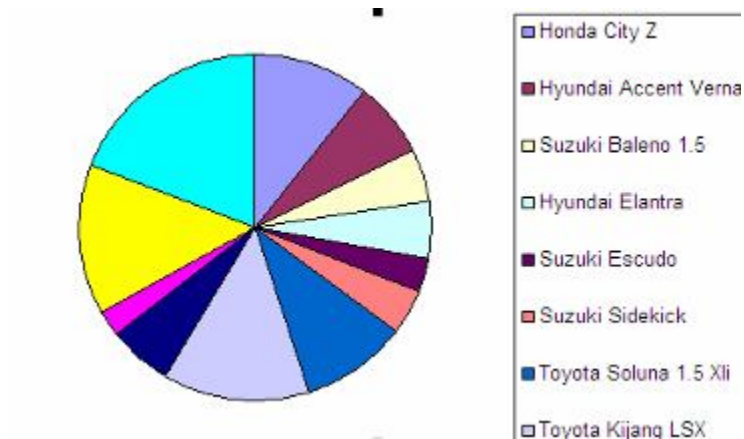
Gambar 36. Grafik pie
