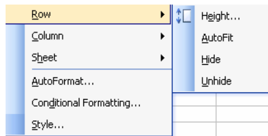
Gambar 31. Menu “Row”
